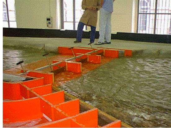
Politecnico di Milano. Vista da monte della traversa e dell'opera di presa nella versione definitiva
